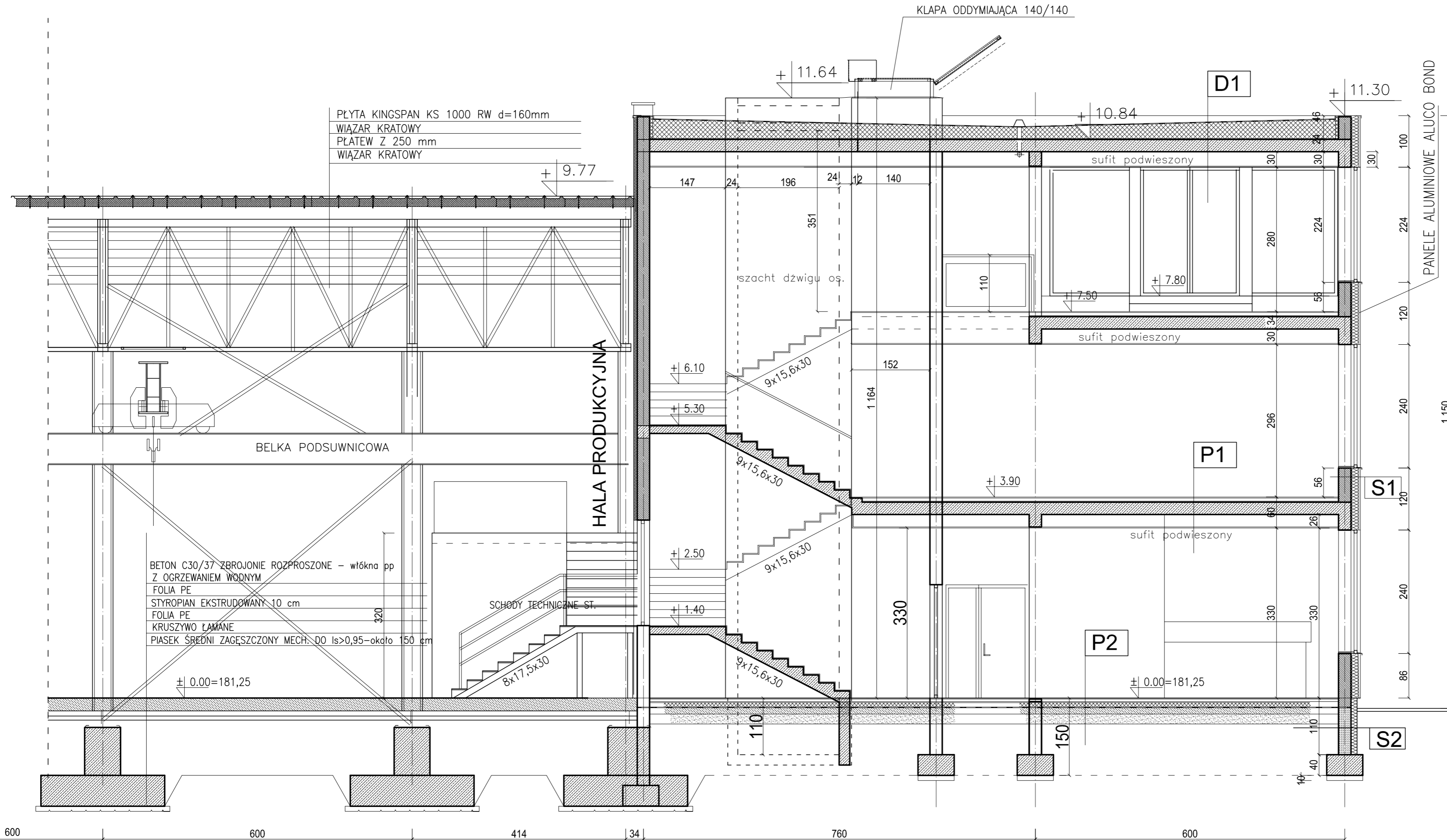
PRZEKRÓJ A-A S 1:50
